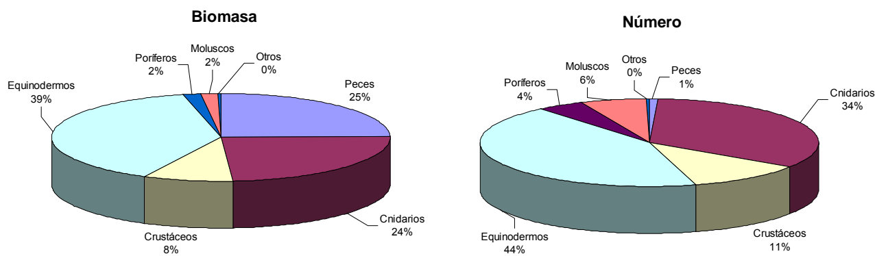
Figura 54. Composición faunística epibentónica en biomasa y número de ejemplares de las muestras de bou de vara
