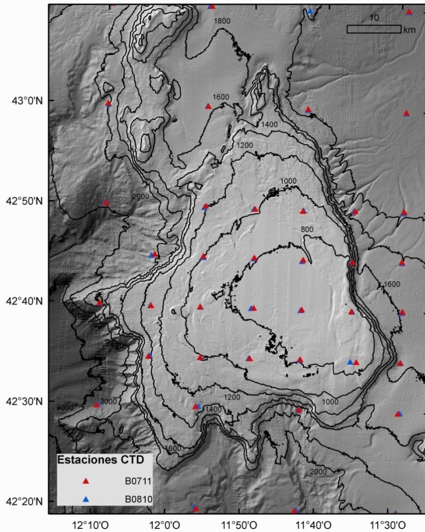
Figura 7. Posiciones de las estaciones hidrográficas
