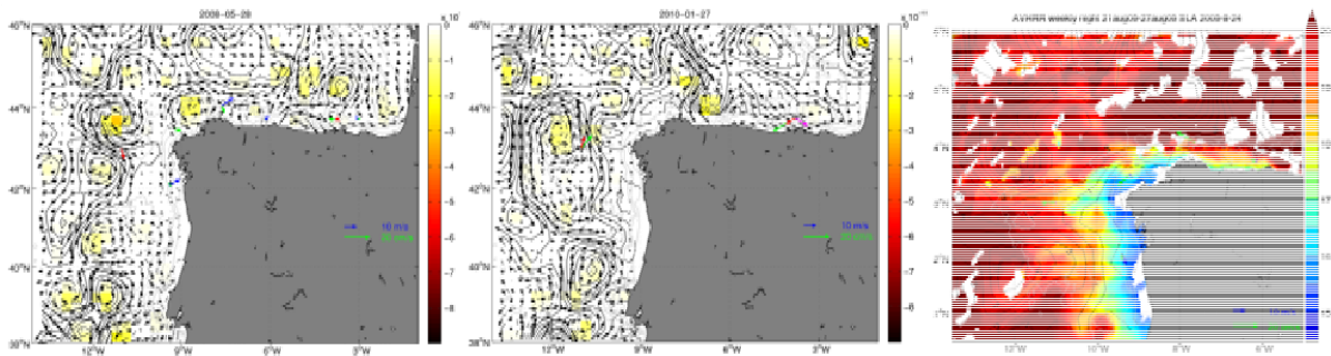
Figura 29.- Campos de corrientes geostóficas (izquierda y centro) mostrando los efectos topográficos producidos por el banco. Filamento de afloramiento que alcanza el banco (derecha). Proyecto VACLAN (IEO).
