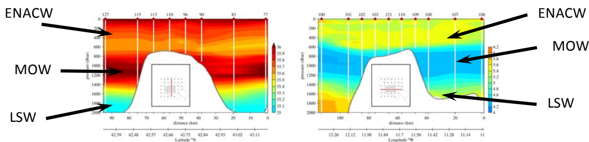
Figura 28.- Izquierda: Sección vertical de salinidad a lo largo de una sección meridional que cruza el eje principal del banco en agosto de 2010. Derecha: Oxígeno disuelto (ml/l) a lo largo de una sección zonal que cruza el eje principal del banco. Se muestran mapas con las isobatas de 1000 y 2000 m y las secciones. Se muestran las capas de agua citadas en el texto. Proyecto VACLAN/COVACLAN- IEO
