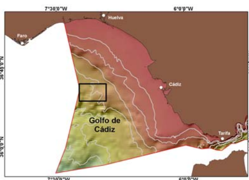
Figura 1. Situación del campo de volcanes de fango de El Laberinto en el Golfo de Cádiz. Lo constituye un conjunto de, al menos, seis volcanes de fango ubicados en el entorno de las dorsales diapíricas de Cádiz y Guadalquivir (Medialdea et al. , 2009).
