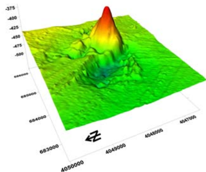
Figura 2. Imagen 3D realizada a partir de datos obtenidos con la sonda multihaz, en la que se puede apreciar la morfología del volcán de fango Gazul, así como los relieves con formas globulares que circundan el cono principal junto a una depresión de colapso. Estos relieves consisten en restos de arrecifes de diversos corales ( Lophelia y Dendrophilia principalmente) que están actualmente extinguidos, encontrándose únicamente algunos pólipos dispersos de tamaño reducido. Acompañan a los arrecifes grandes enlosados calcareníticos y chimeneas carbonatadas.
