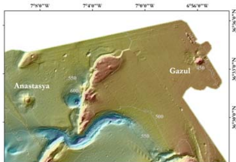
Figura 3. Localización del volcán de fango Gazul en relación con los que componen el campo de El Laberinto (Anastasya, Pipoca y Tarsis). Se comprueba que Gazul es el más somero de los descubiertos hasta la fecha.
