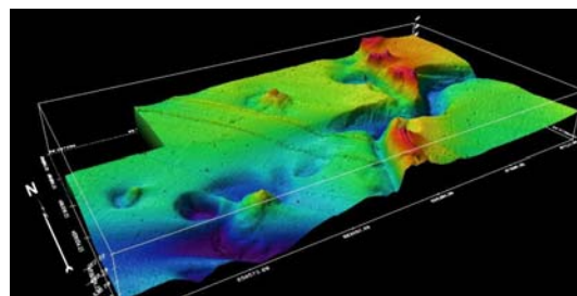
Figura 4. Imagen 3D realizada a partir de datos obtenidos con la sonda multihaz, en la que se observan los tres volcanes submarinos más importantes de los que componen el campo de El Laberinto (Anastasya, Pipoca y Tarsis).
